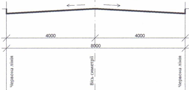
Поперечний профіль січення 1-1 М 1:100
